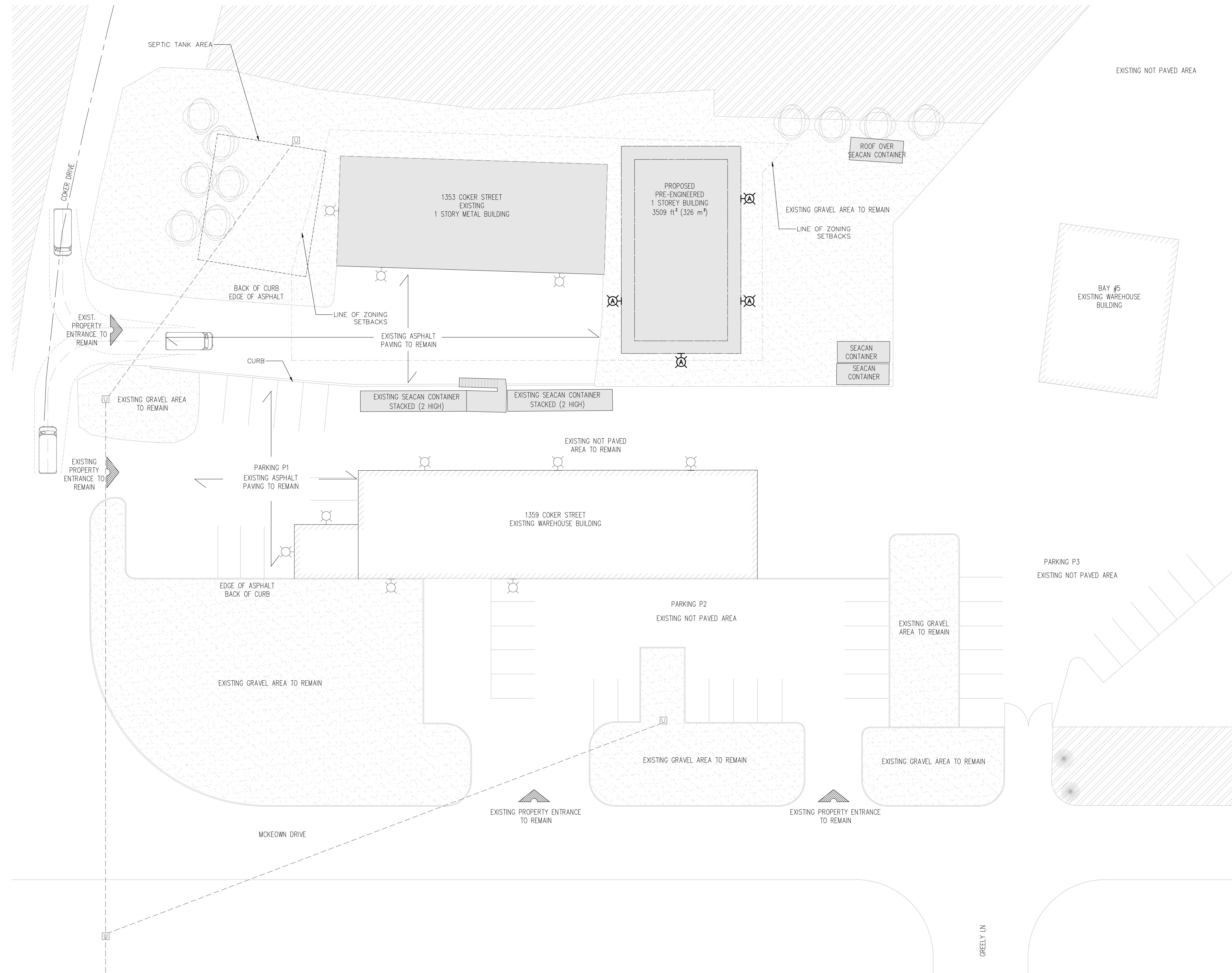
1 ELECTRICAL SITE PLAN E004 1:250
