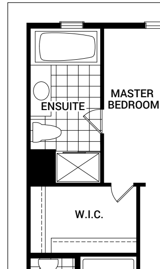
OPTIONAL ENSUITE LAYOUT A
