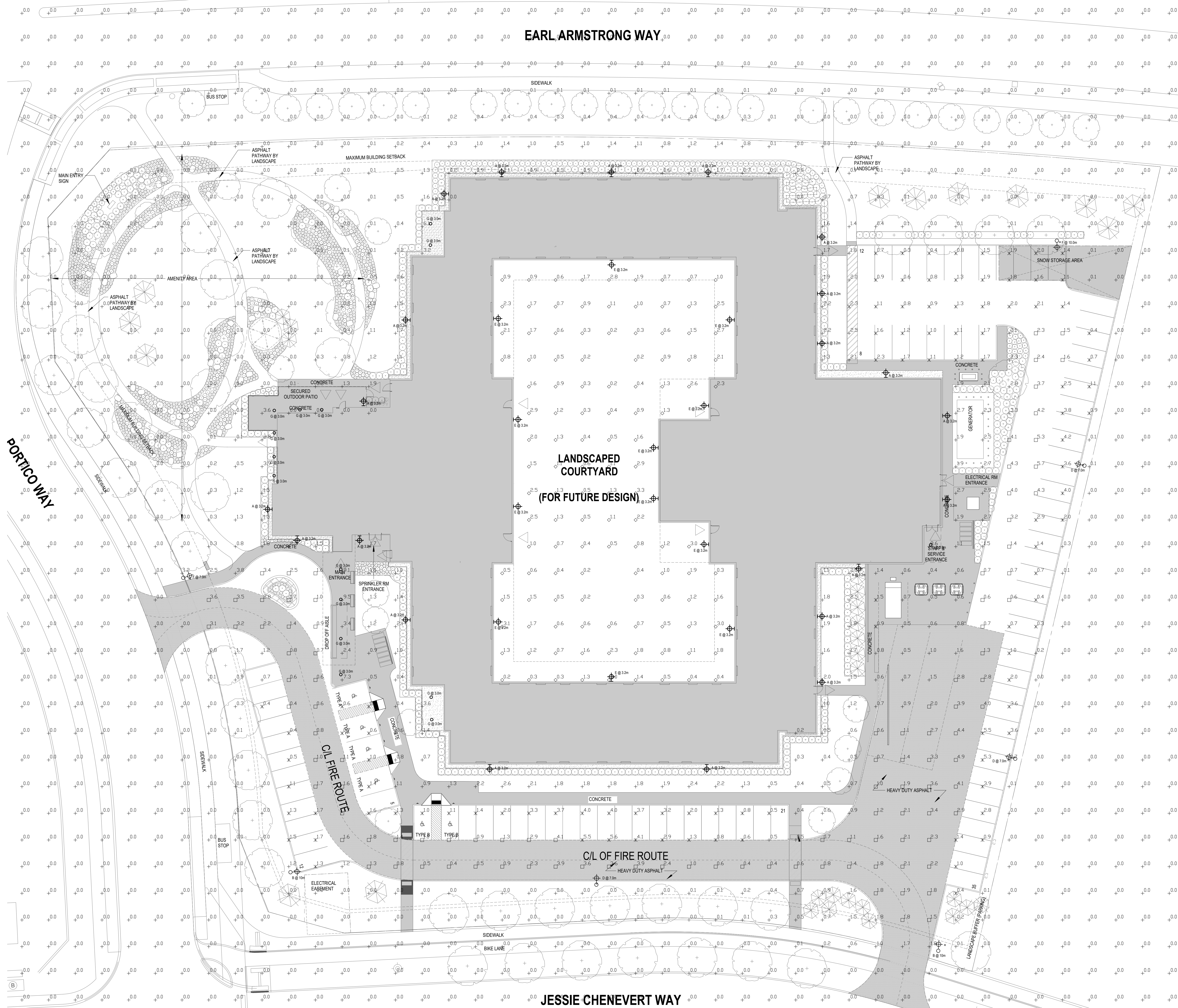
1 SITE PLAN PHOTOMETRICS E-102 1/200
