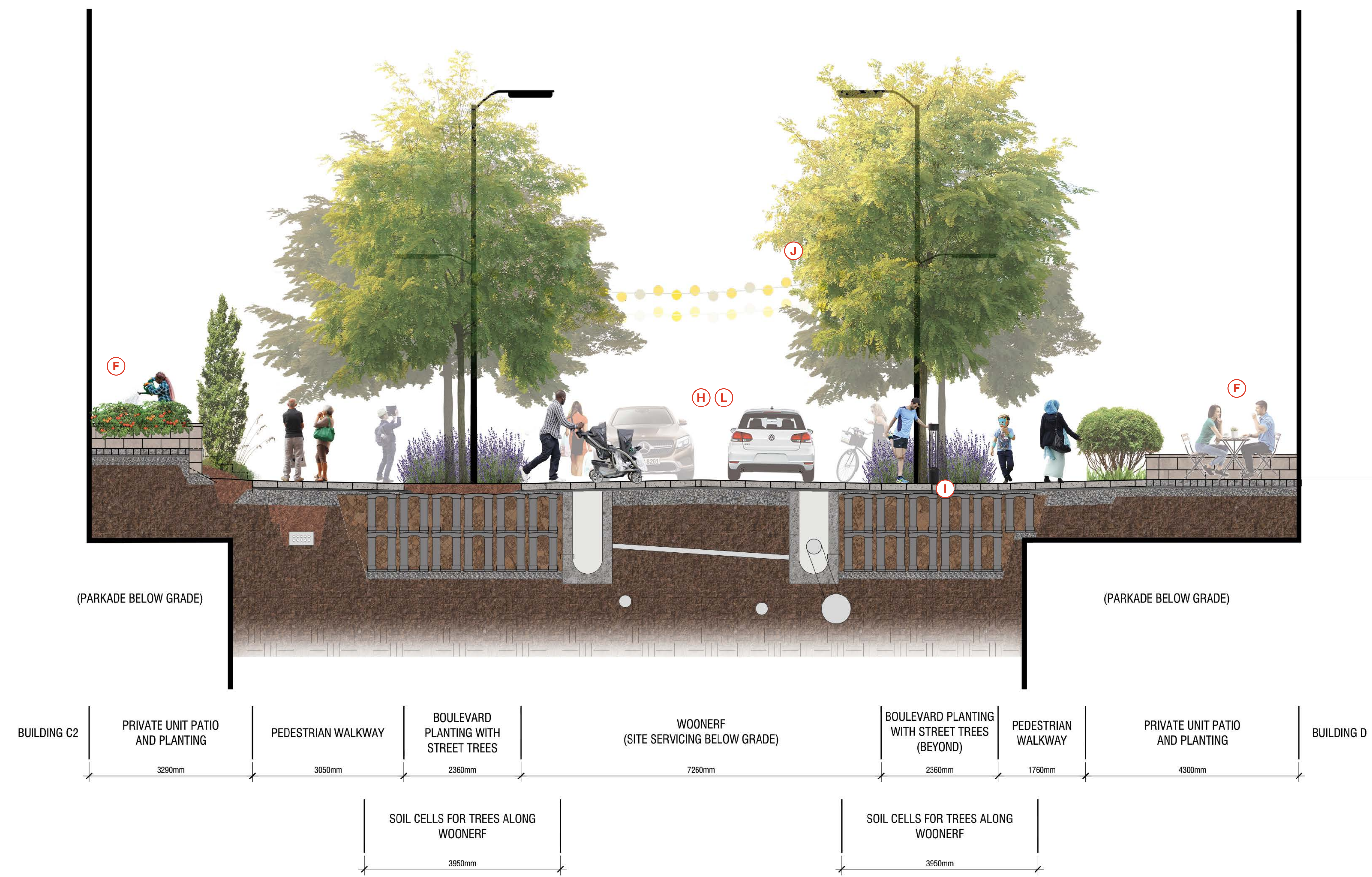
1 SECTION A-A AT WOONERF L2 1:50
