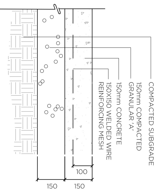
5 CONCRETE PAVEMENT N.T.S. L-02
