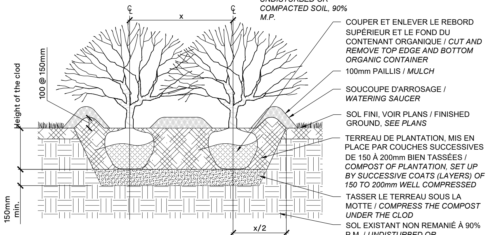
PLANTATION D'ARBUSTES / SHRUB PLANTING Échelle / Scale 1:20
