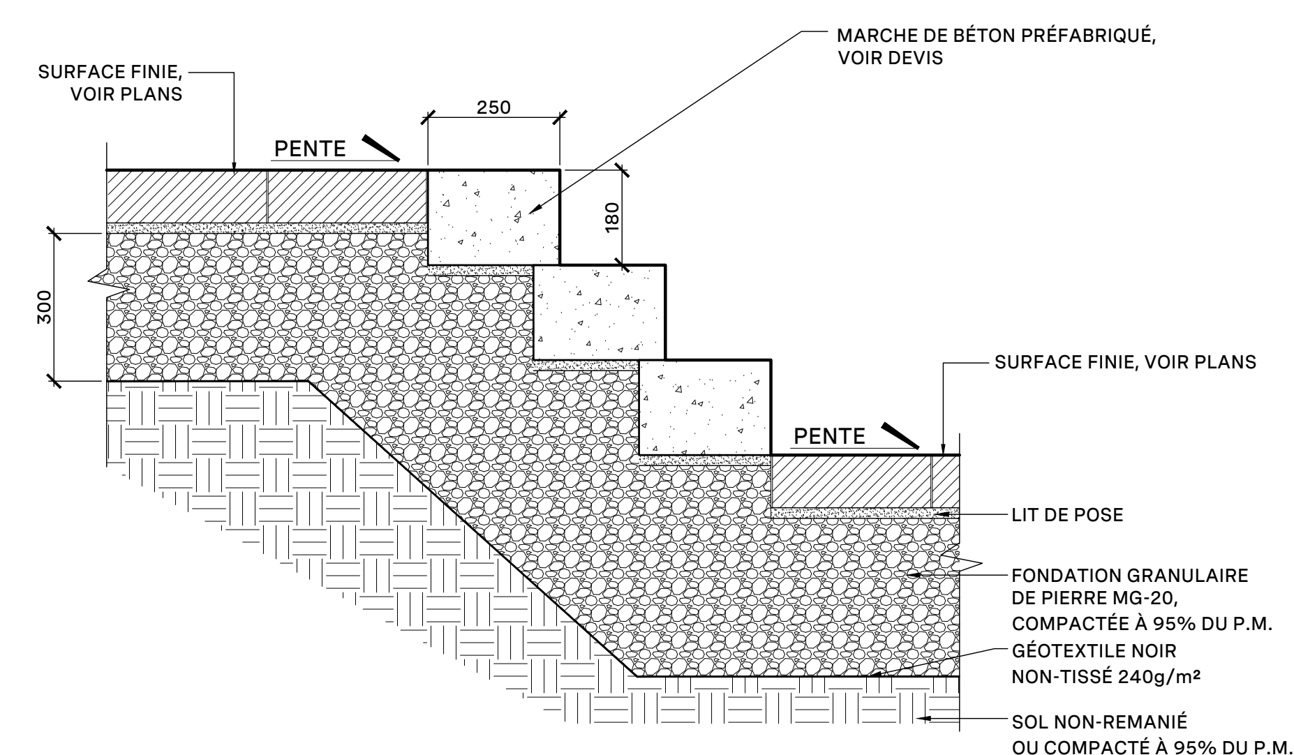
50 MARCHE DE BÉTON PRÉFABRIQUÉ Échelle 1:10
