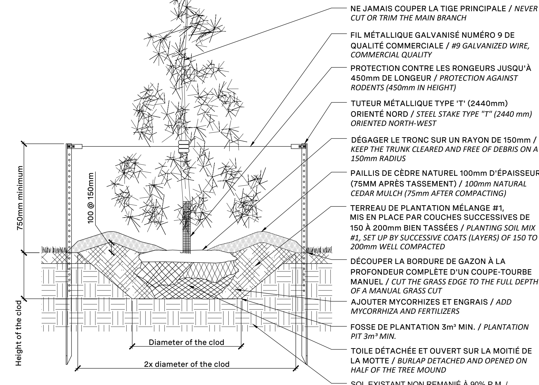
PLANTATION D'ARBRES CONIFÈRE / CONIFEROUS TREE PLANTING Échelle / Scale 1:20
