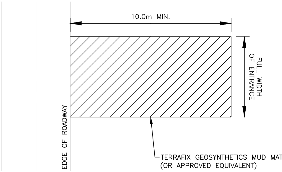
MUD MAT DETAIL N.T.S.
