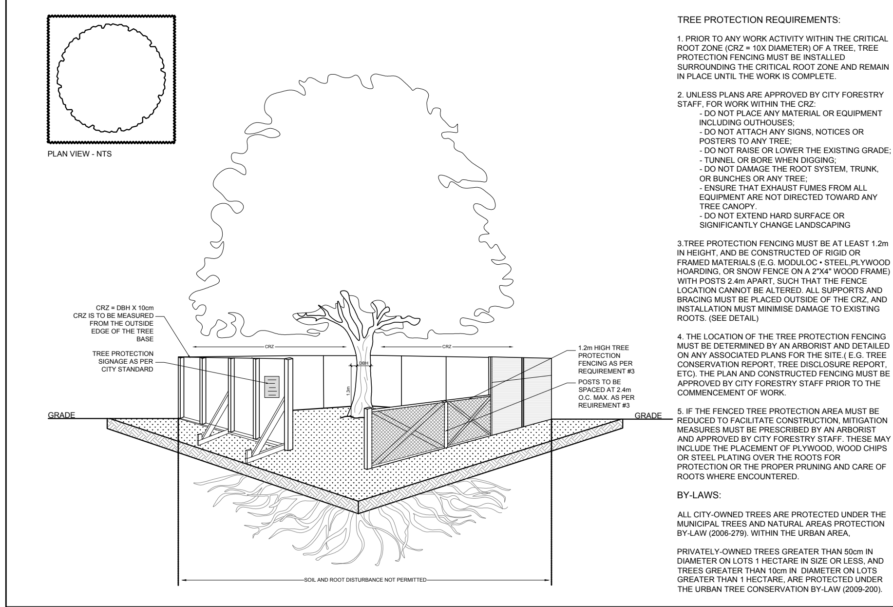
2 TREE PROTECTION FENCING TCR SCALE: N.T.S.
