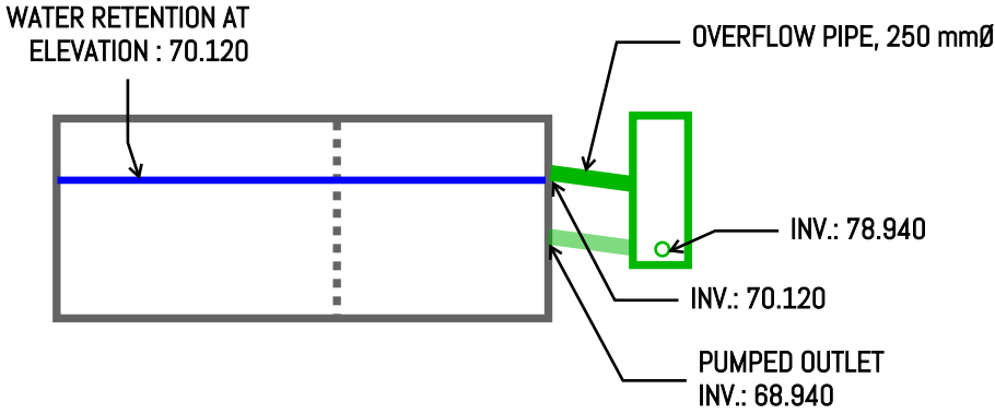
PROFIL VIEW
