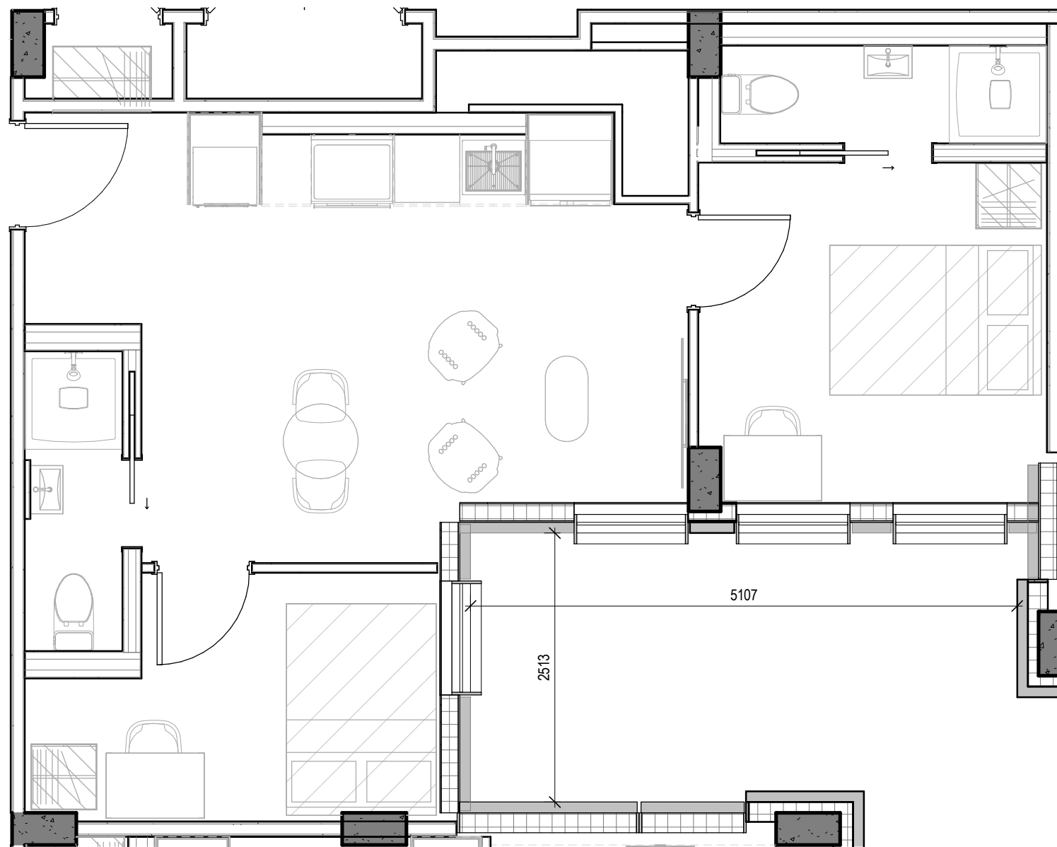
1 A906 2 BEDROOMS - UNIT 475, 375, 276, 174
