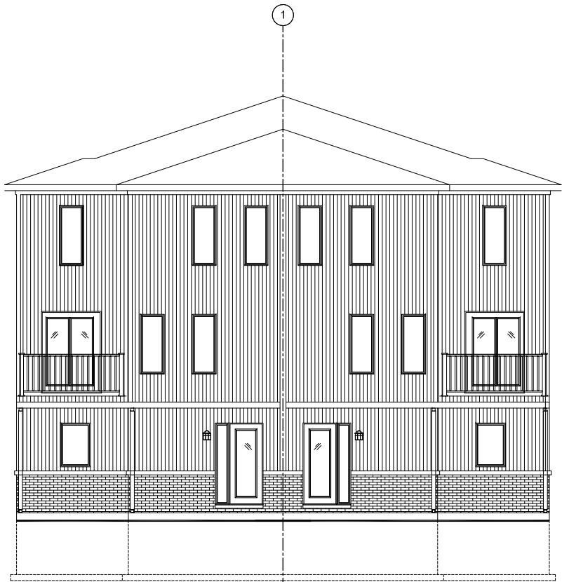
BB-3 ELEV. 'E' (REV.) CORNER
