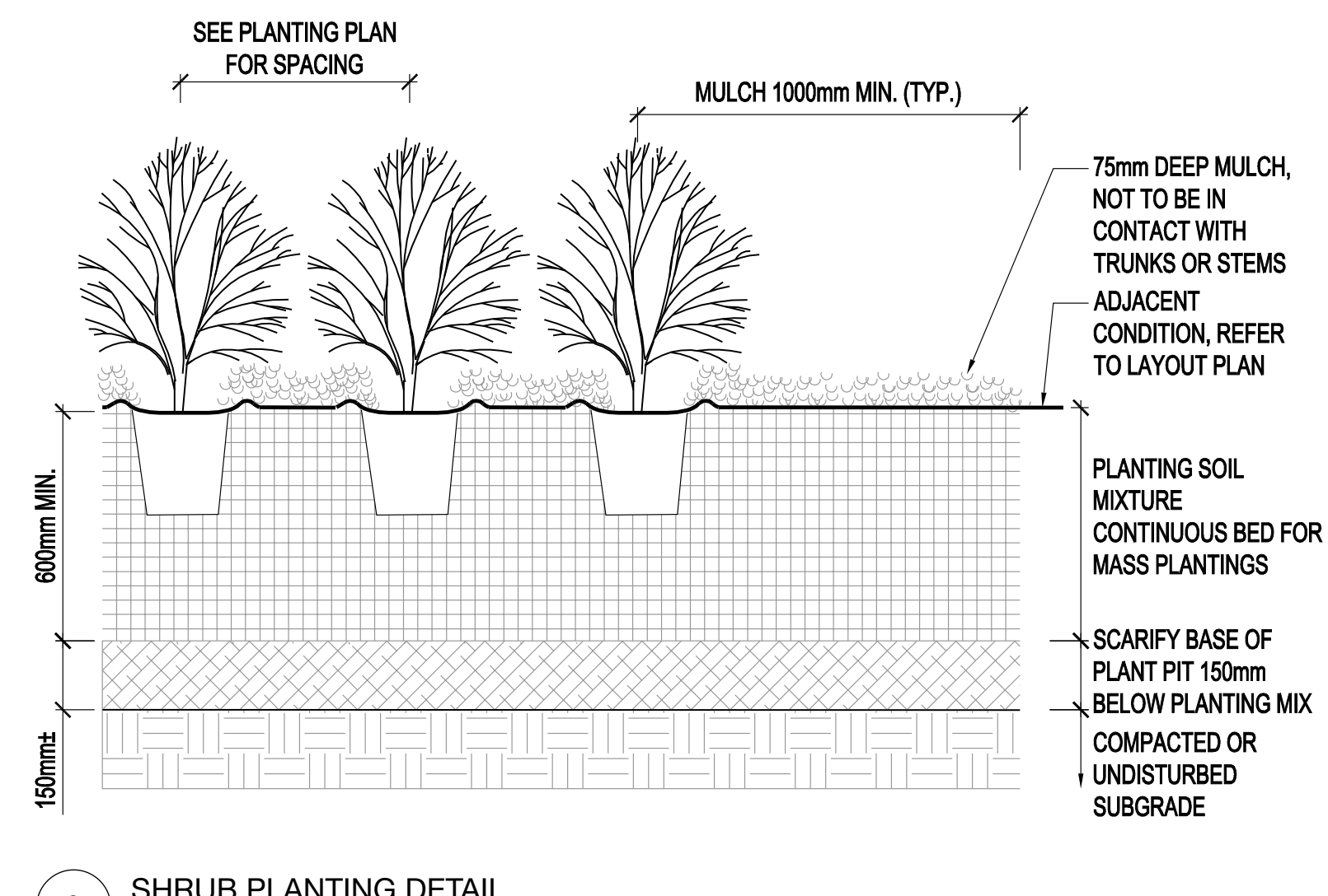
9 SHRUB PLANTING DETAIL Scale: N.T.S.
