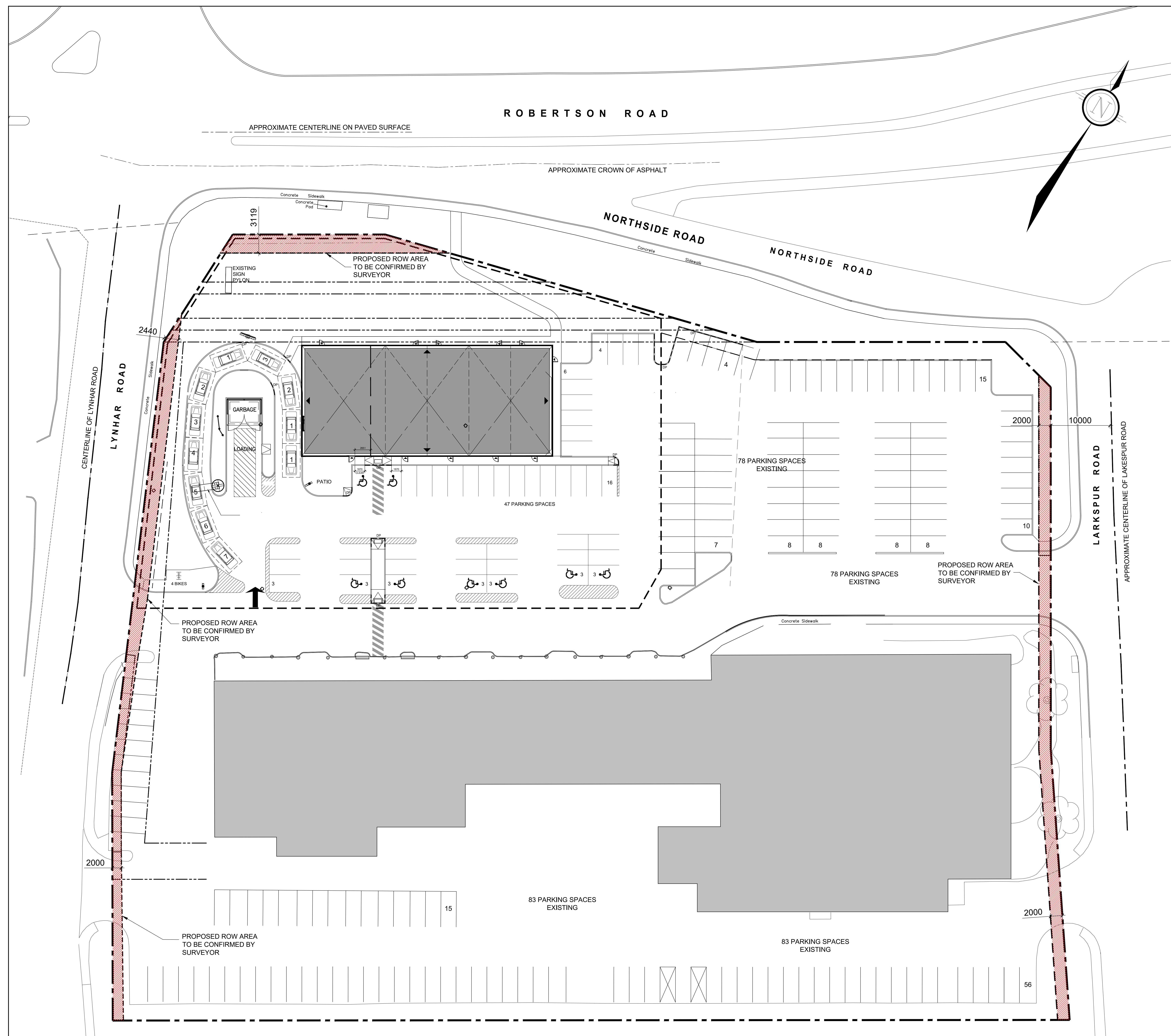
1 ROW PROTECTION PLAN SP-A02 SCALE: 1:250
