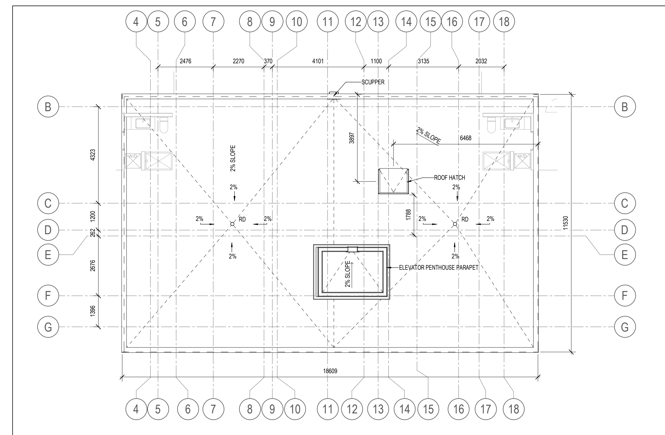
1 T.O. UPPER ROOF A107 SCALE: 1 : 100
