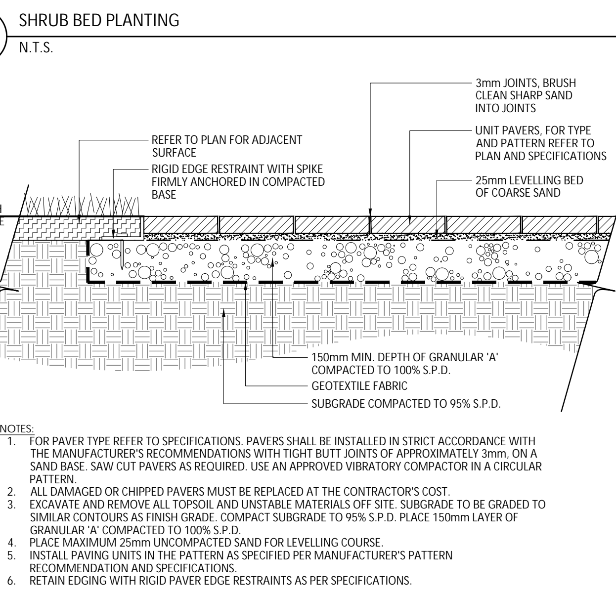
3 PEDESTRIAN UNIT PAVING N.T.S.
