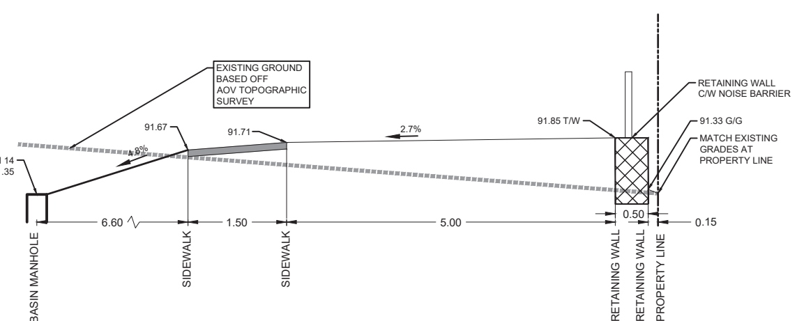
DETAIL B-B N.T.S.
