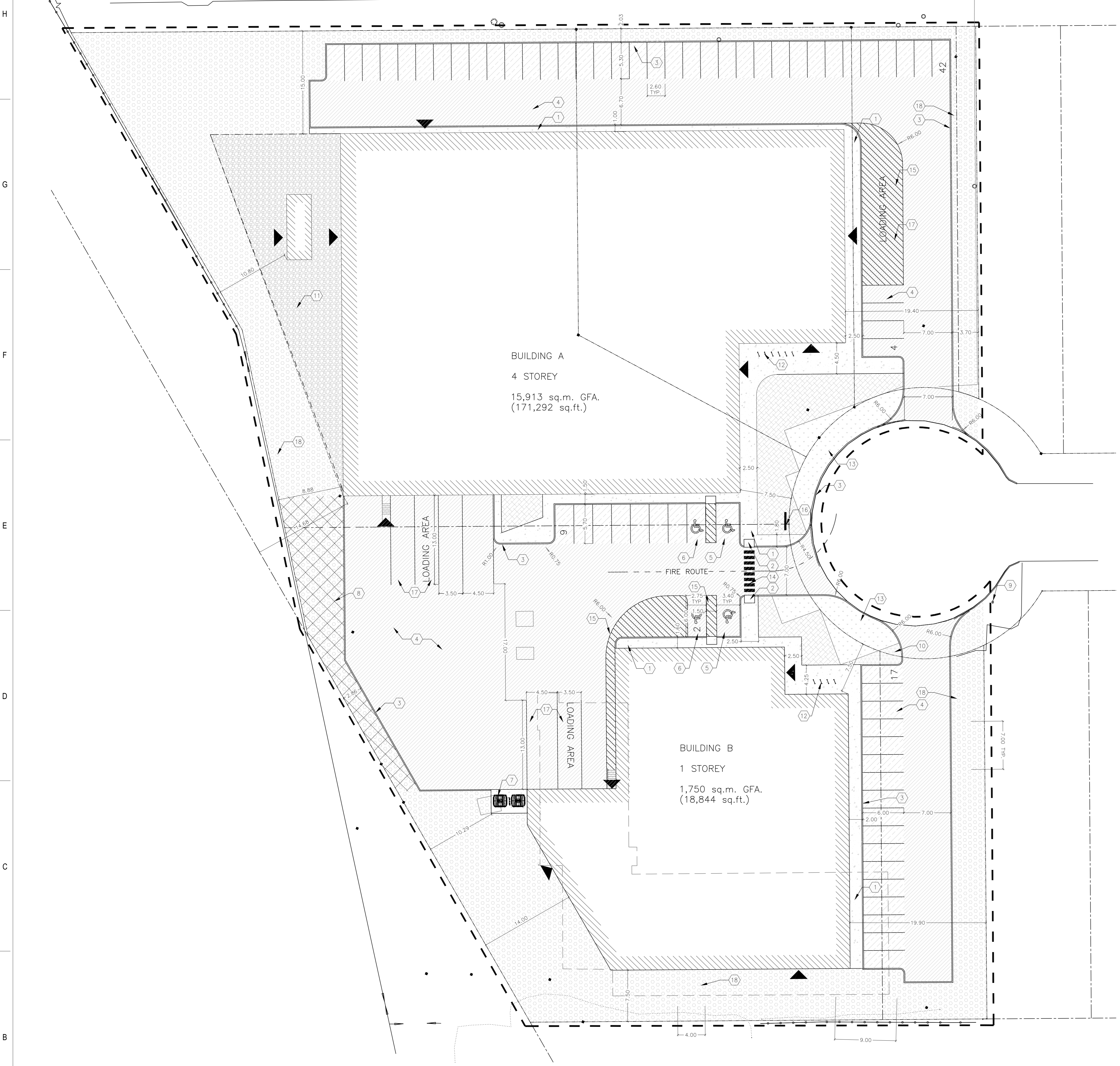
1 SITE PLAN L100 1:250
