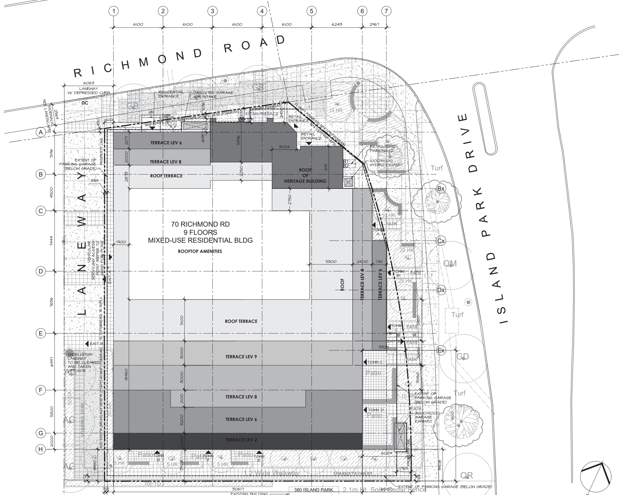
1 SITE PLAN A1.01 1:125
