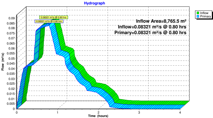
Link 2L: Ditch
