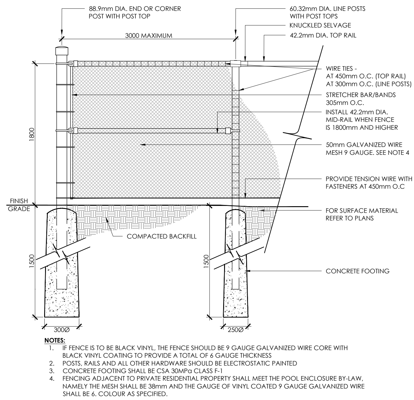
2 1.8m CHAINLINK FENCE N.T.S.
