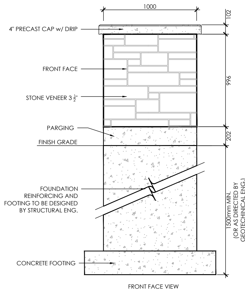
4 COLUMN ENTRY FEATURE N.T.S.
