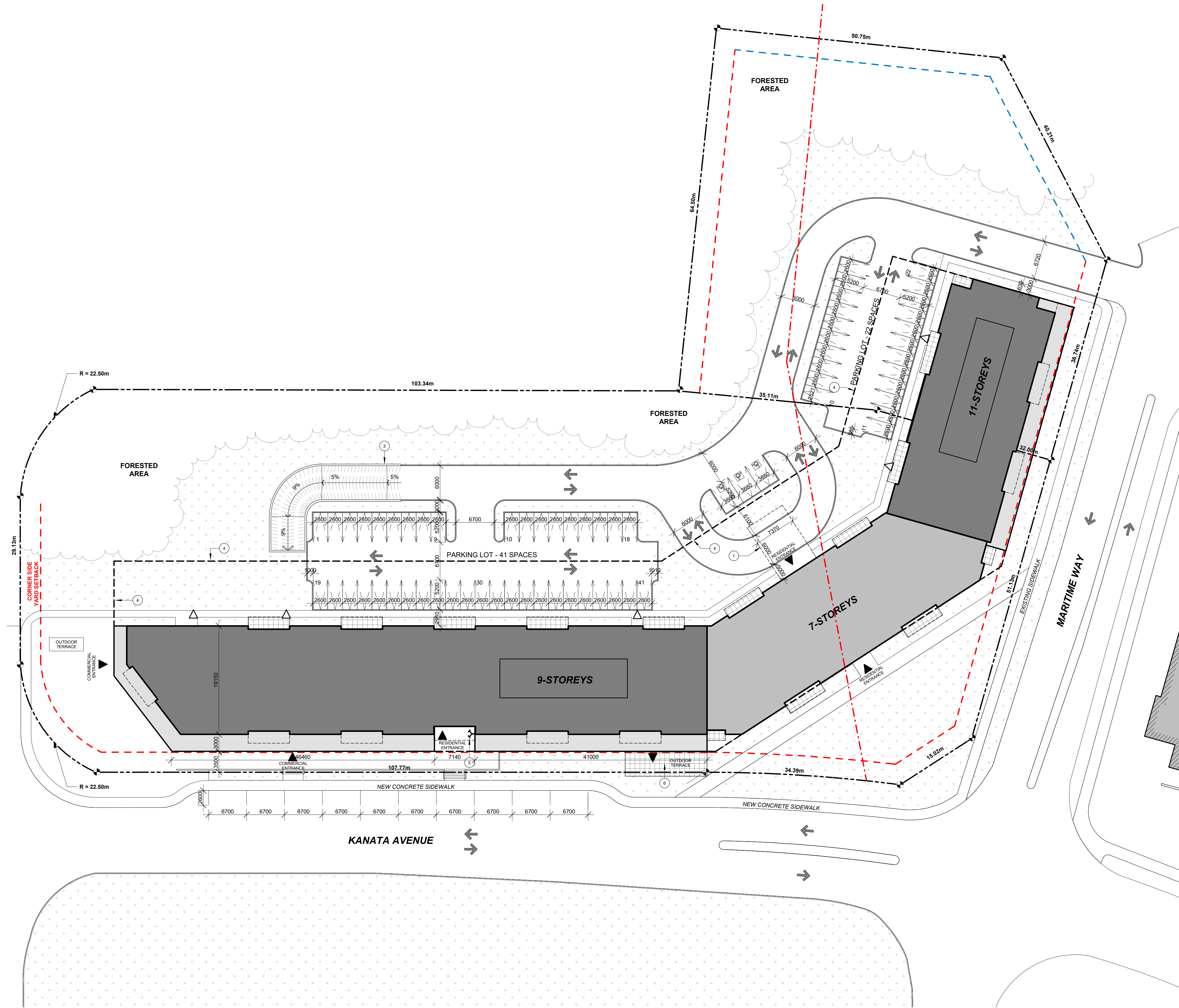
1 SITE PLAN 1 : 350
