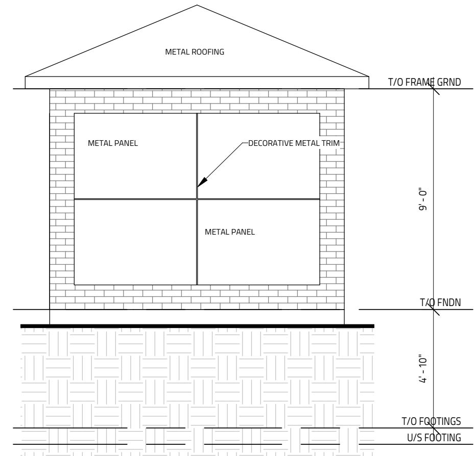
2 RIGHT ELEVATION SCALE: 1/4" = 1'-0"
