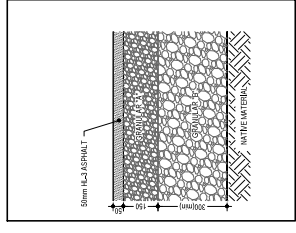
3 LIGHT DUTY ASPHALT SCALE: N.T.S.
