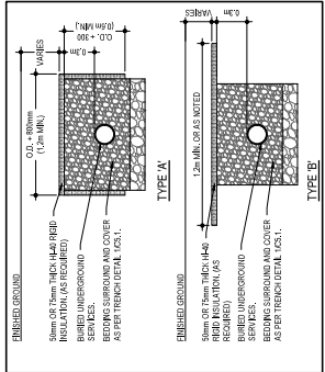
1 FROST PROTECTION DETAIL SCALE: N.T.S.
