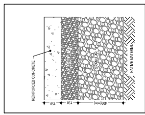
2 CONCRETE PAD STRUCTURE SCALE: N.T.S.
