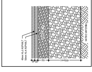
4 HEAVY DUTY ASPHALT SCALE: N.T.S.
