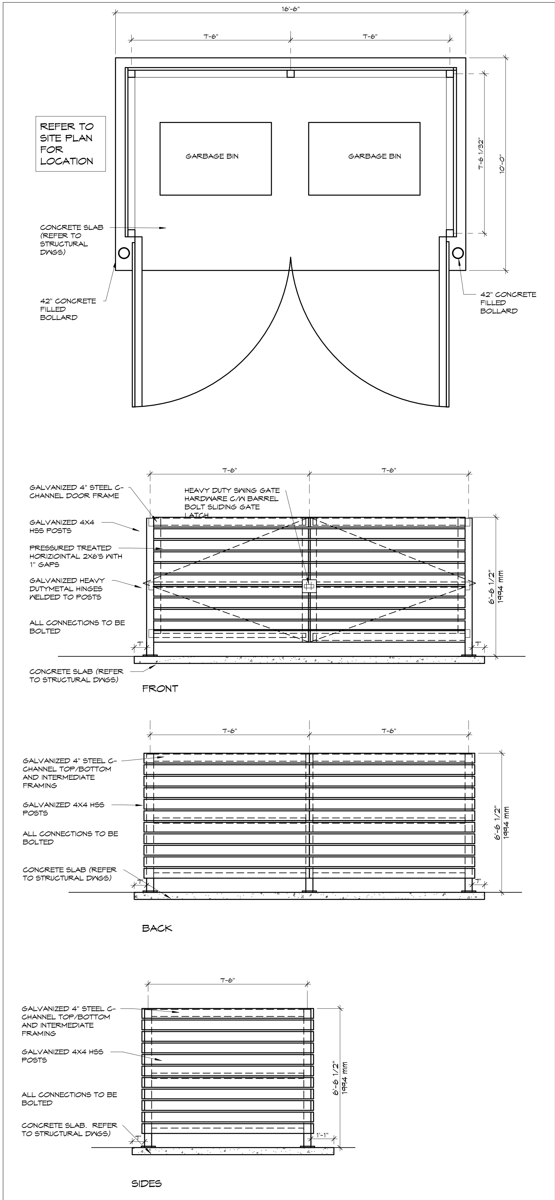
1 A3 / SCALE: 3/8" = 1'-0"
