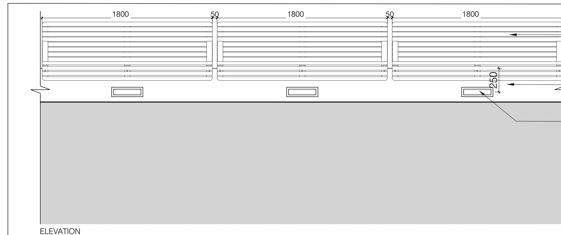
ELEVATION
