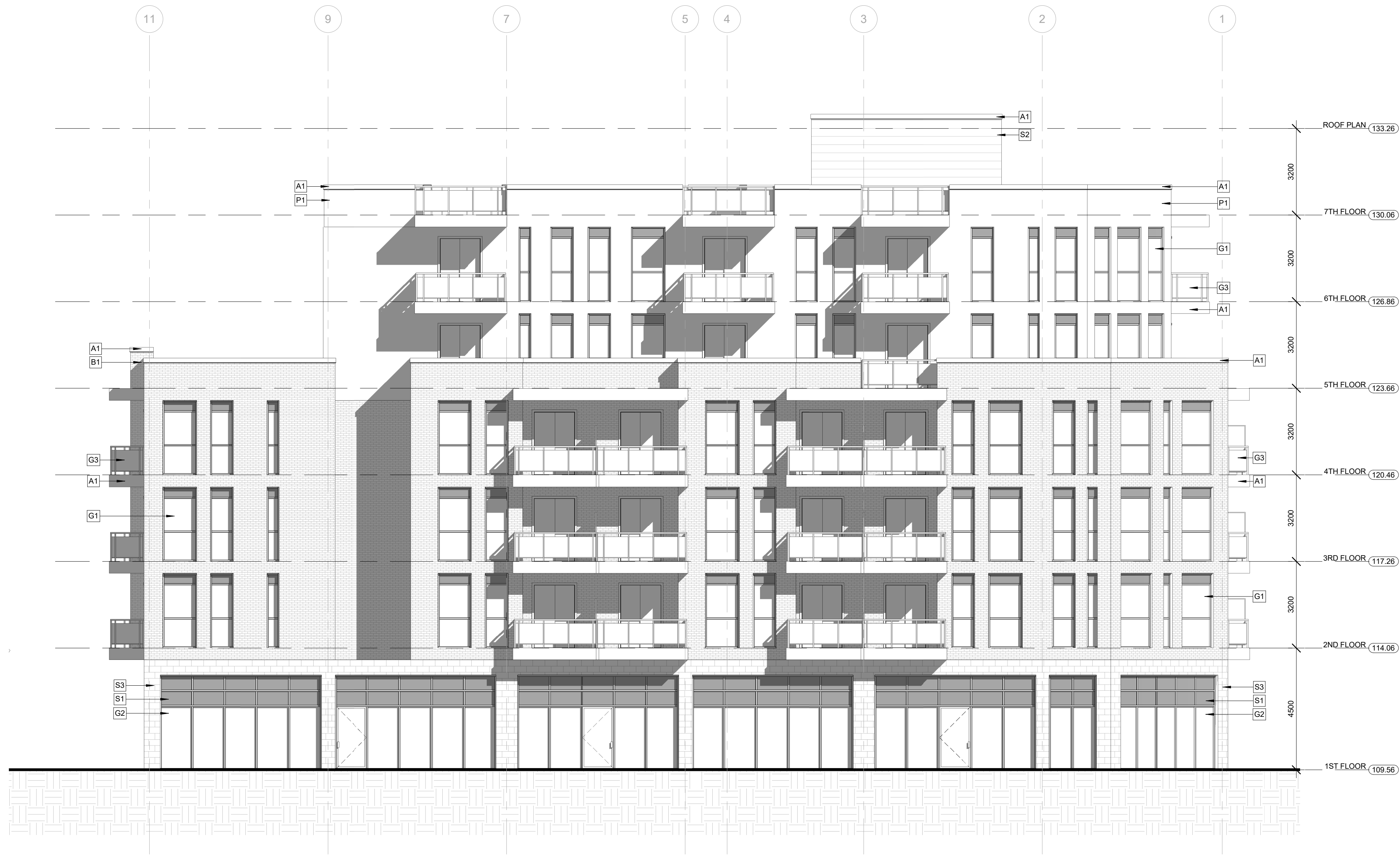
2 C West C407 Scale: 1 : 100
