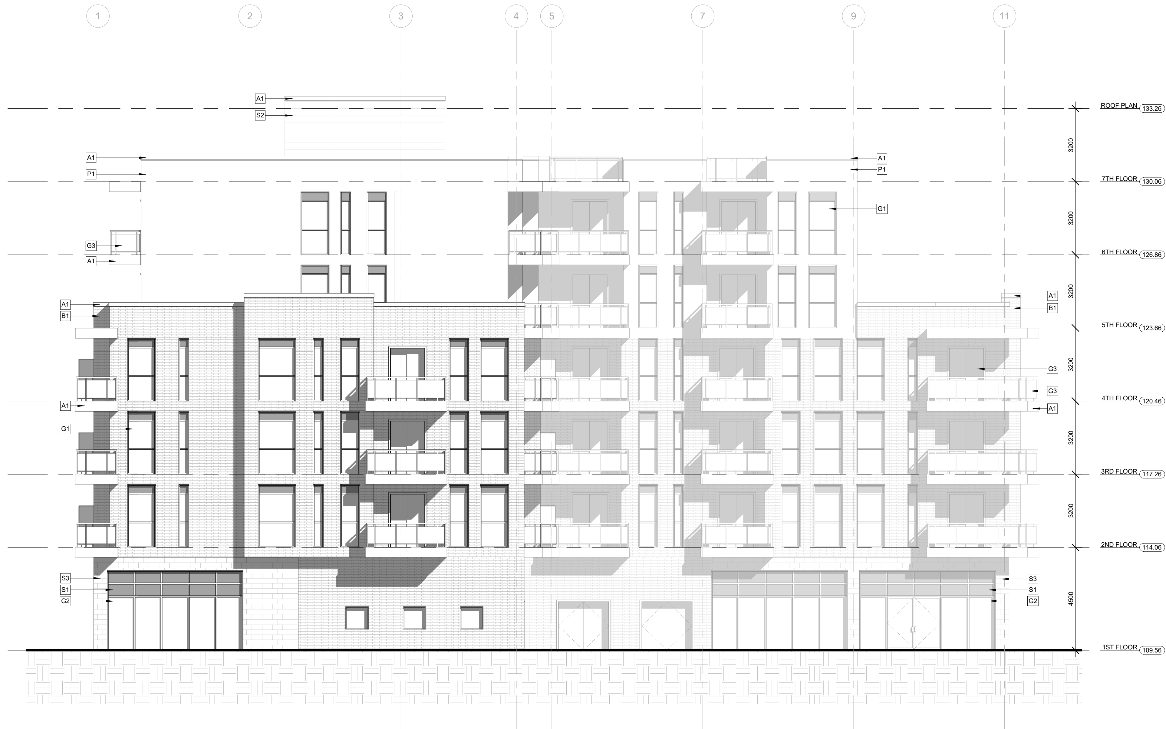
1 C East C407 Scale: 1 : 100
